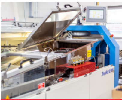
SEHO-Powerwave Wellenlötautomat
